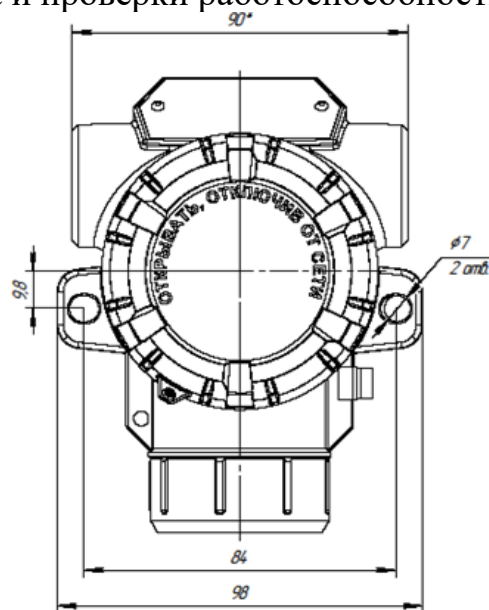
Рисунок 34 - Монтажные размеры
